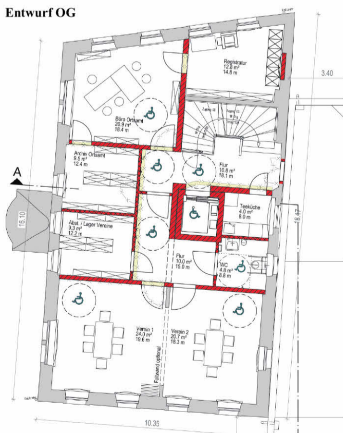
Entwurf OG
