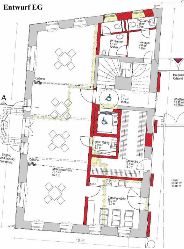
Entwurf EG
